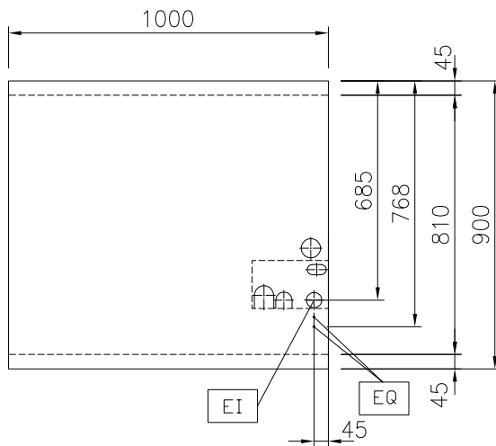
Planta
